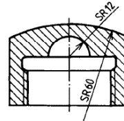
Figure 7: Standard representation UNE 1-039-94
